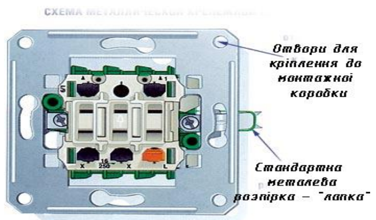
Схема металевої кріплячої пластини
