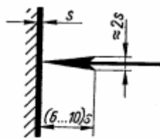
Розміри елементів стрілки.
