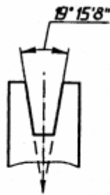
Умовне позначення кутового розміру.
