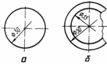
Нанесення неповної розмірної лінії розміру діаметра: a — при повному зображенні кола; б — при частковому зображенні кола.
